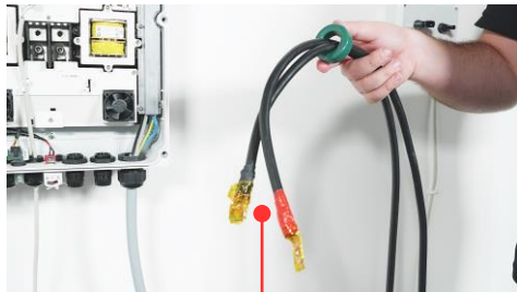
Schrumpfschlauch
